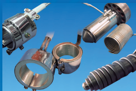
ノズルヒーター
